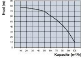
Performans Eğrisi 9LD925-2 R 626
