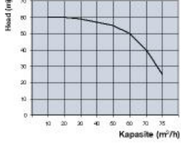
Performans Eğrisi 12 LD 477 - 2C 65 A
