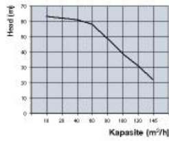
Performans Eğrisi 9LD925-2 R 822
